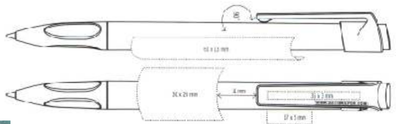
Article: 2645 ANTIBAC, stylo a bille rétractable - zones d'impression
